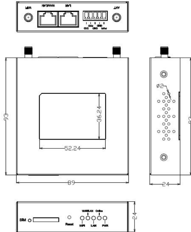
导轨安装路由器尺寸
