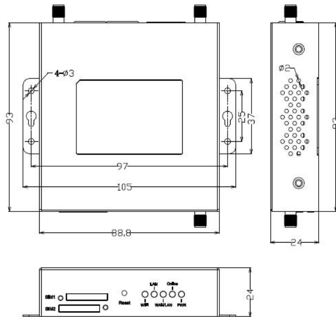
耳架安装路由器尺寸
