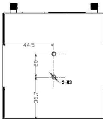
导轨安装位置
